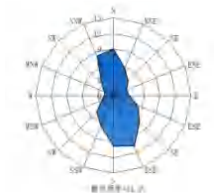
图 3.1-3 鄄城县风向玫瑰图
